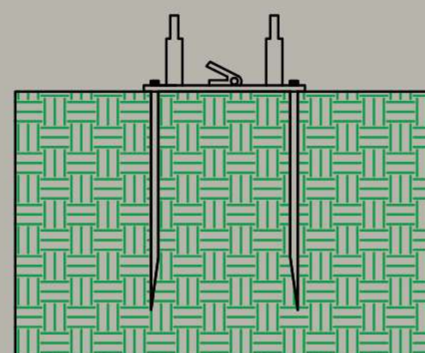
ESTACADO A PISO
