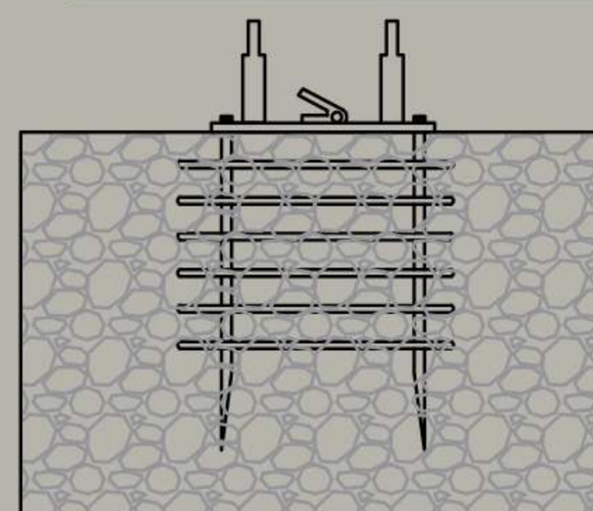
FUNDACIÓN DE HORMIGÓN
